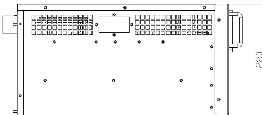
图 2-10 ANSVG-100kvar 模块机箱侧视图
