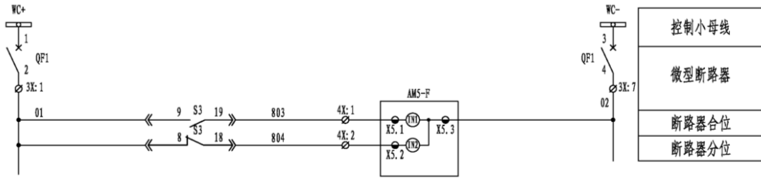
图 5.3 开入回路接线方法
