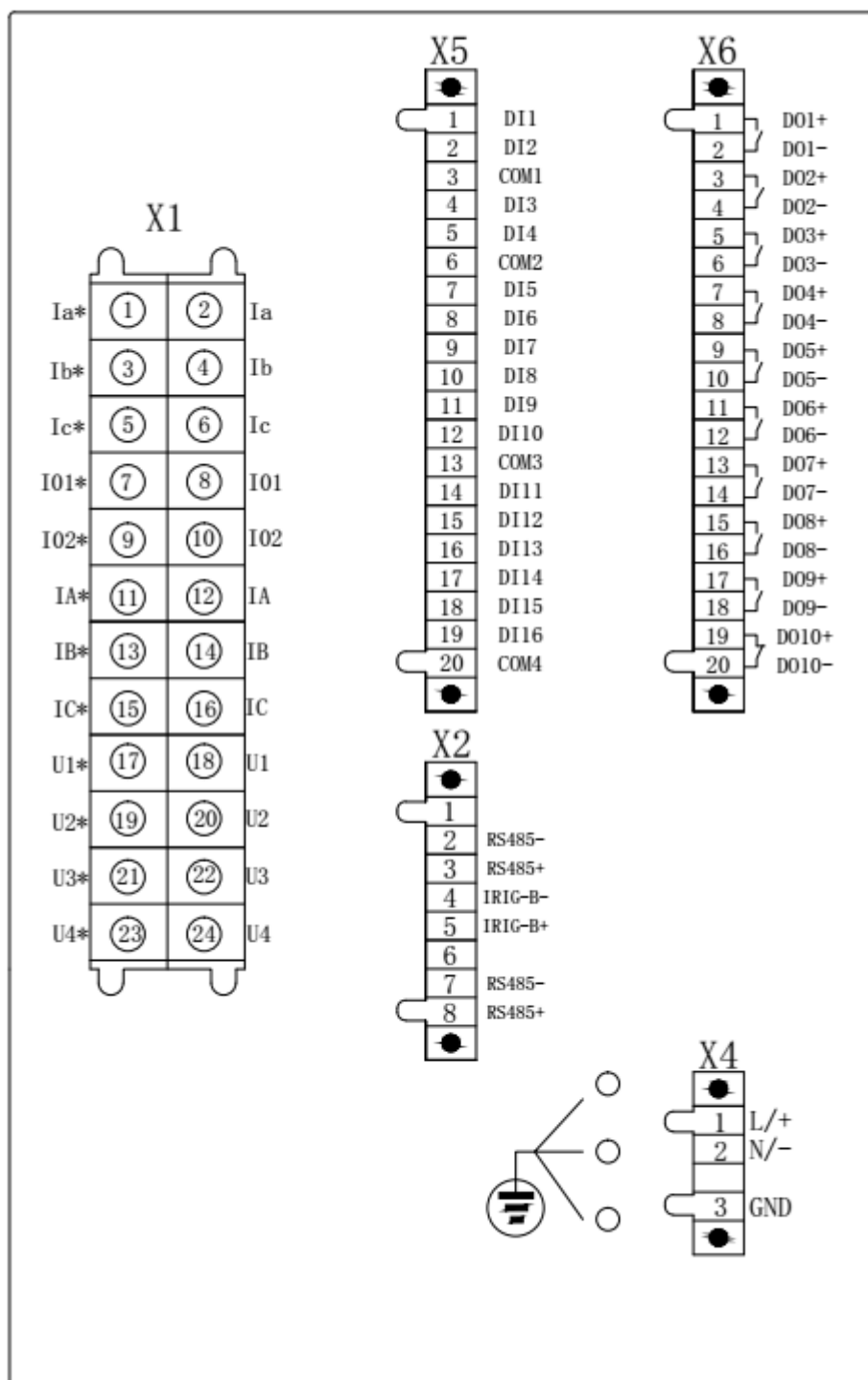
图 5.1 装置电气接线图
