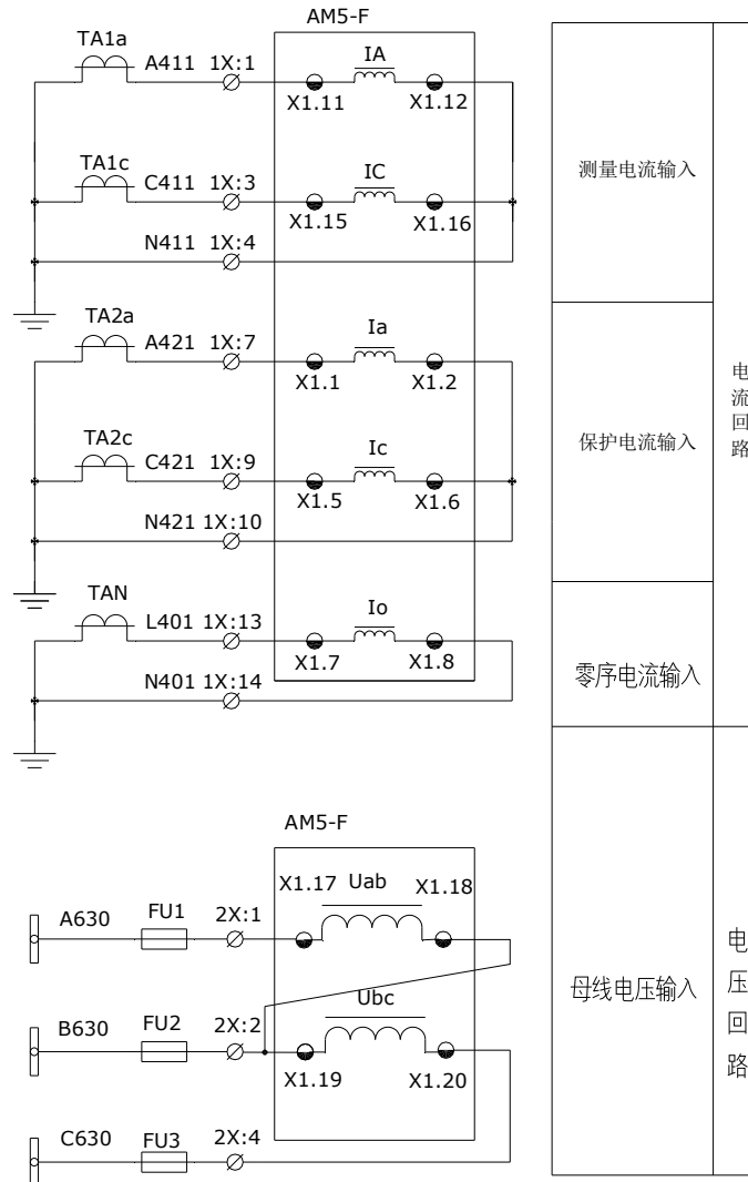
图 5.2 2PT 2GT 接线方法
